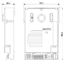
Zeichnung Dimensionen
