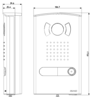
Zeichnung Dimensionen
