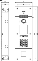
Zeichnung Dimensionen
