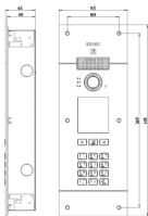
Zeichnung Dimensionen
