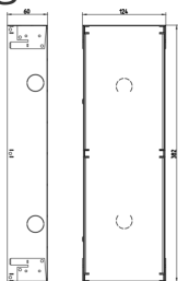
Zeichnung Dimensionen
