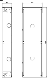
Zeichnung Dimensionen
