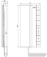
Zeichnung Dimensionen
