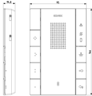
Zeichnung Dimensionen
