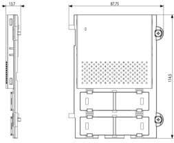
Zeichnung Dimensionen
