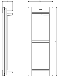
Zeichnung Dimensionen
