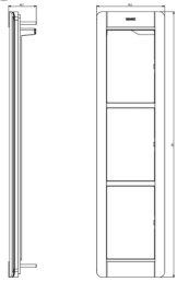
Zeichnung Dimensionen
