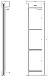
Zeichnung Dimensionen
