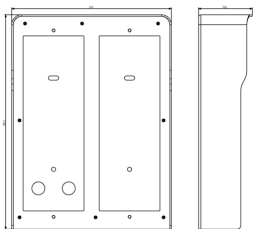
Zeichnung Dimensionen
