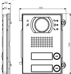
Zeichnung Dimensionen
