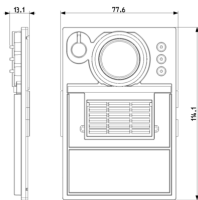
Zeichnung Dimensionen
