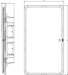
Zeichnung Dimensionen
