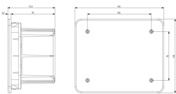
Zeichnung Dimensionen
