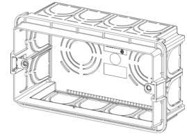
3D-Ansicht
