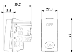
Διαστάσεις
