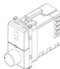
3d σχέδιο
