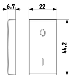
Διαστάσεις
