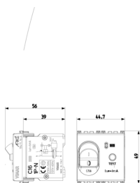
Διαστάσεις
