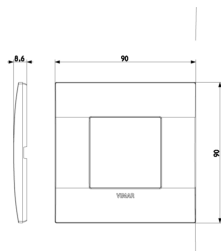
Διαστάσεις
