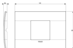
Διαστάσεις
