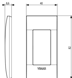
Διαστάσεις
