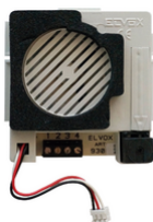
930B - Μον. ήχου Sound System σύνδ. δύο καλωδ.
