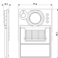
Διαστάσεις
