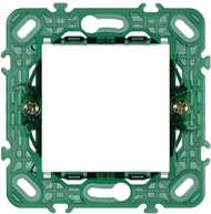
14602 - Soporte 2M + garras eje 71mm
