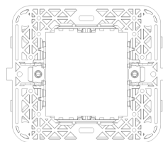
Vista trasera
