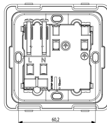
Vista trasera
