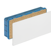
V70008 - Caja derivación empotrable 391x154x70mm
