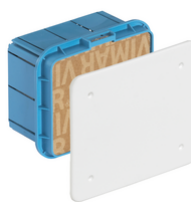
V70003 - Caja derivación empotrable 116x92x70mm
