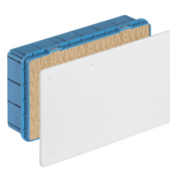
V70007 - Caja derivación empotrable 287x154x70mm
