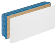
V70010 - Caja derivación empotrable 515x201x80mm
