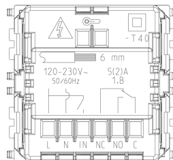
Vue arrière
