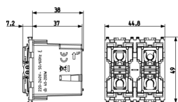
Dessin dimensions hors-tout
