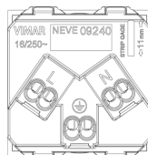
Vue arrière
