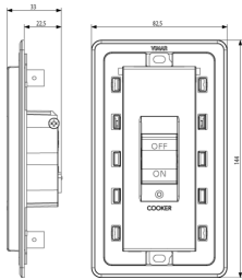
Dessin dimensions hors-tout
