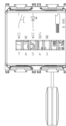
Vue arrière
