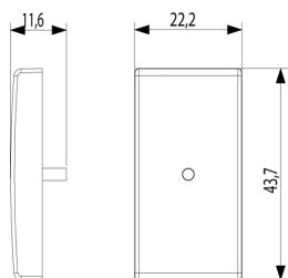
Dessin dimensions hors-tout
