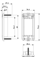
Dessin dimensions hors-tout
