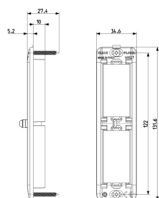
Dessin dimensions hors-tout
