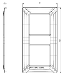
Dessin dimensions hors-tout
