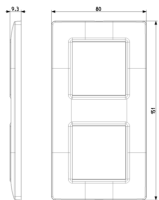
Dessin dimensions hors-tout
