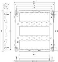
Dessin dimensions hors-tout
