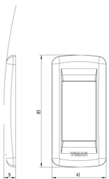
Dessin dimensions hors-tout
