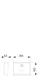
Dessin dimensions hors-tout
