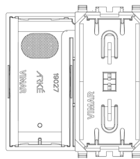
Vue arrière
