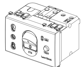
Dessin 3D
