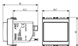
Dessin dimensions hors-tout
