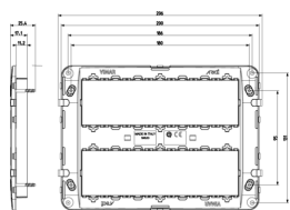
Dessin dimensions hors-tout
