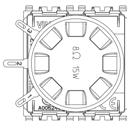
Vue arrière
